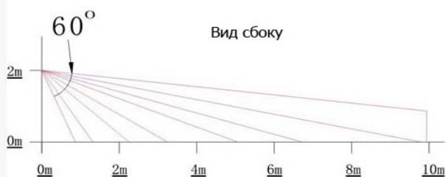
Зона охвата датчика движения
